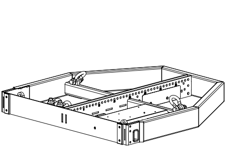
Z5300 J Flugrahmen Für bis zu vierundzwanzig J8/J12 Lautsprecher oder vierzehn J Subwoofer
