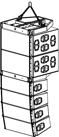
Gemischtes J-Serie Array mit 2 x Z5300 J Flugrahmen Z5303 J Sicherungskettensatz
