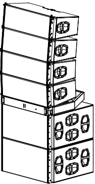
J-Serie Groundstack mit Z5300 J Flugrahmen
