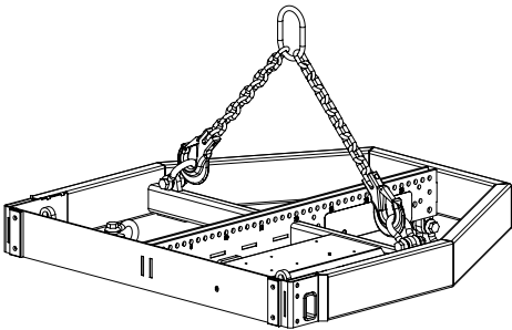
Z5300 J Flugrahmen Lieferumfang: Z5303 J Sicherungskettensatz 2 x J Lastadapter 2 x J Front Links 2 x Locking Pinsets 10 mm 1 x Locking Pinset 11 mm 1 x Montageplatte für SSE® ProSight oder Rieker® Neigungsmesser
