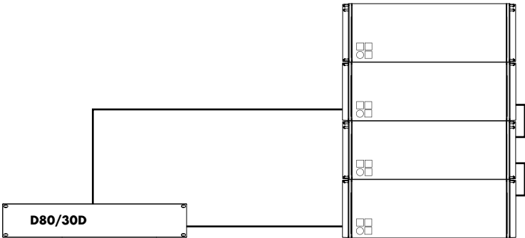
D80/30D Verstärker im 2-Weg-aktiv-Betrieb für J8 und/oder J12
