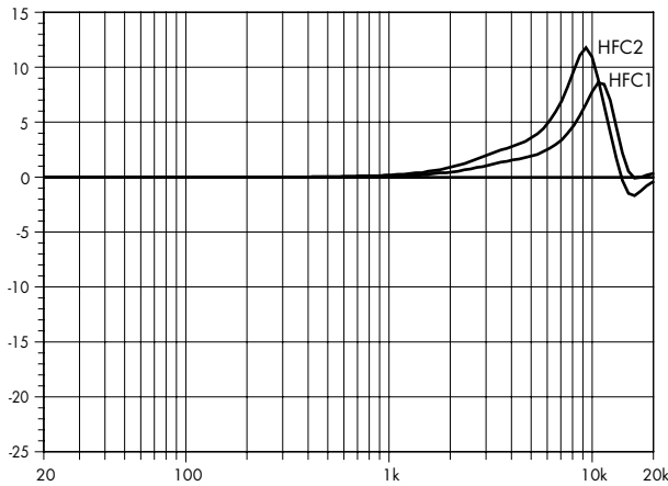
HFC-Korrektur*
