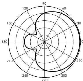
Polardarstellung, Hyperkardioid
