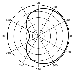
Polardarstellung, Standardkardioid
