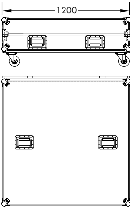
E7441 Touring Case 1 x J Flugrahmen
