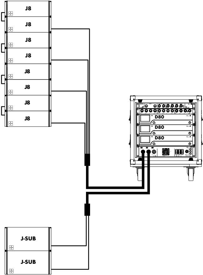
J-Serie Konfiguration mit geflogenem J8 Line-Array und am Boden gestellten J-SUBs mit einem D80 Touring Rack
