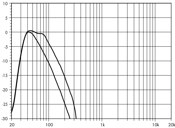
J-SUB Standard und INFRA
