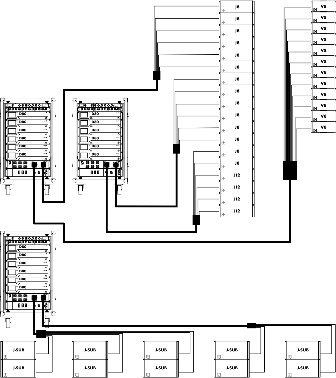
J-Serie Konfiguration mit J8/J12 als Hauptarrays und V8 als Outfills mit ArrayProcessing sowie J-SUBs am Boden mit D80 Touring Racks
