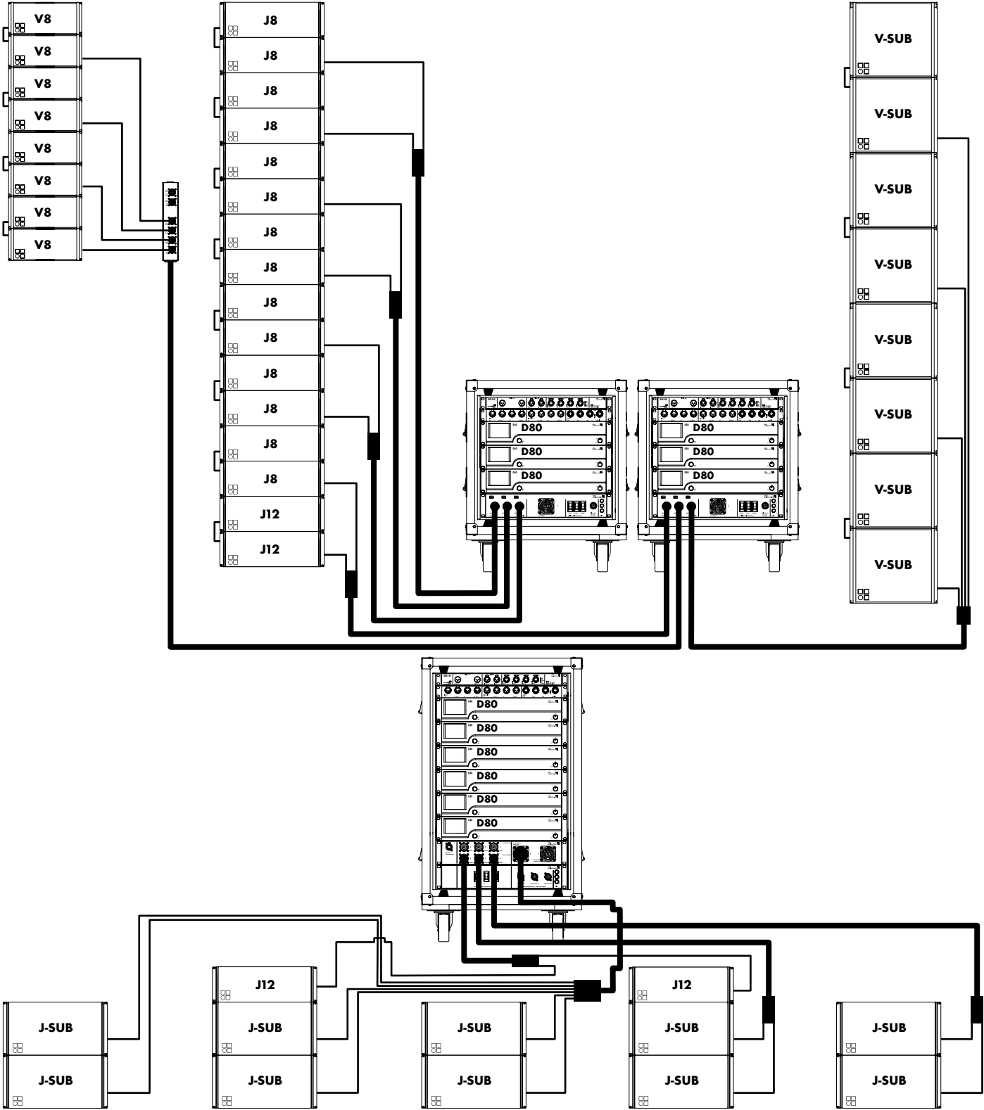
J-Serie Konfiguration mit J8/J12 als Hauptarrays und V8 als Outfills sowie J-SUBs am Boden mit D80 Touring Racks
