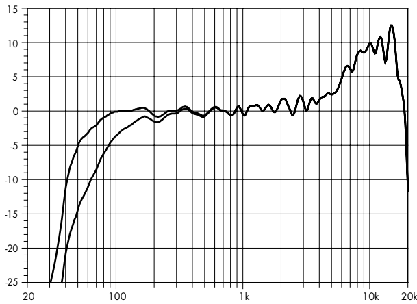
J8 Standard und CUT (einzelner Lautsprecher)
