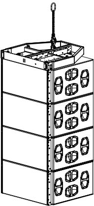
J-SUB Array mit Z5300 J Flugrahmen Z5305 J Anschlagkette
