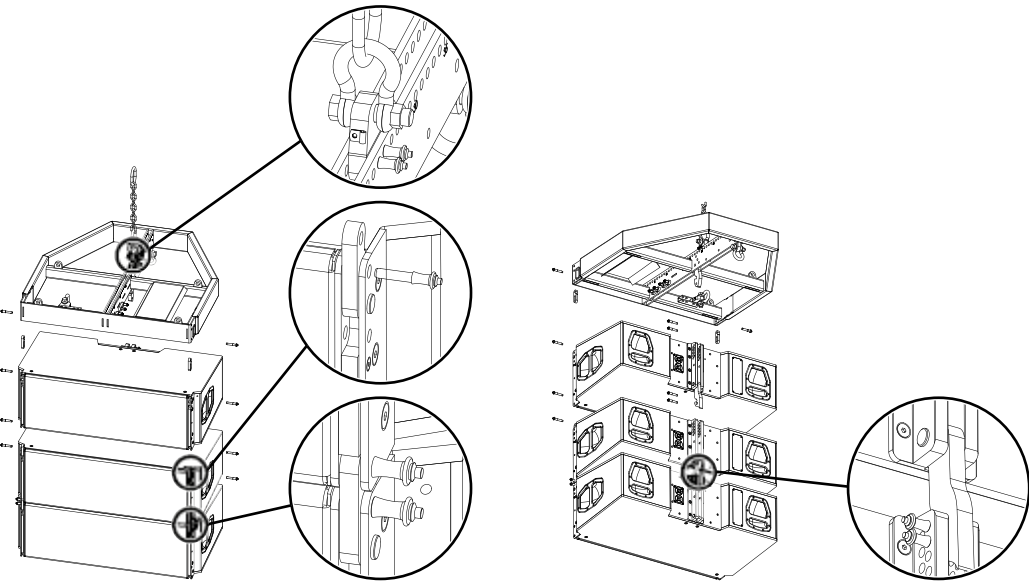
J-Serie Riggingssystem
