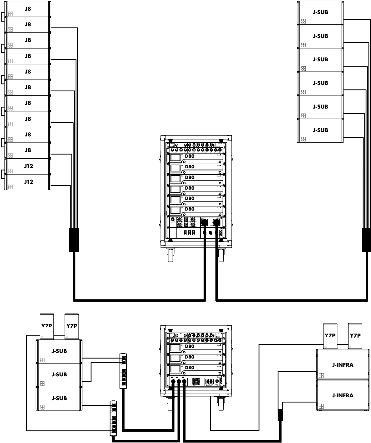
J-Serie Konfiguration mit J8/J12 Hauptarrays, einer geflogenen J-SUB Spalte und J-SUB/J-INFRA am Boden sowie Y7Ps als Nearfills mit D80 Touring Racks.
