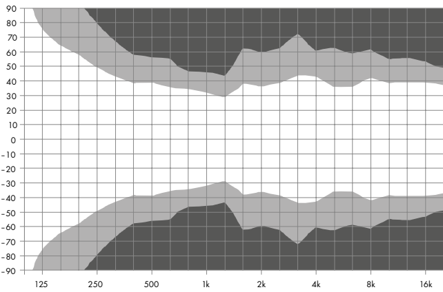
J8 horizontale Abstrahlcharakteristik 2
