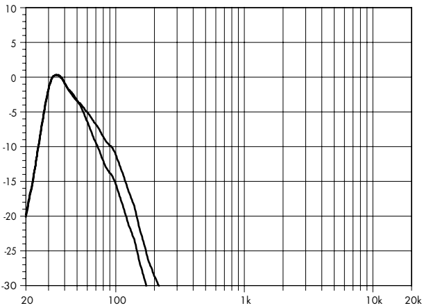
J-INFRA Standard und 70 Hz
