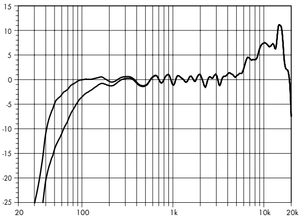
J12 Standard und CUT (einzelner Lautsprecher)
