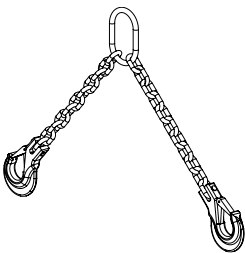
Z5303 J Sicherungskettensatz
