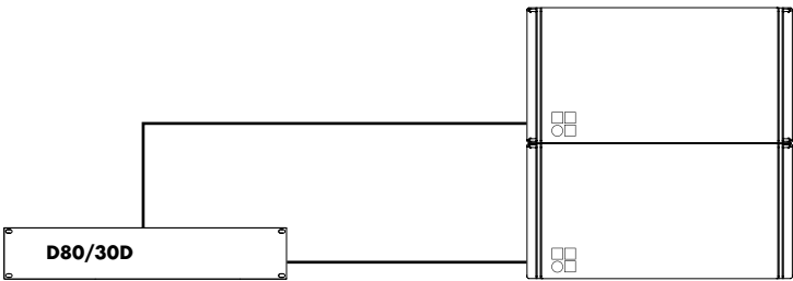
D80/30D Verstärker im 2-Weg-aktiv-Betrieb für J-SUB und/oder J-INFRA
