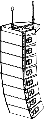
J8/J12 Array mit Z5300 J Flugrahmen 2 x Z5305 J Anschlagkette
