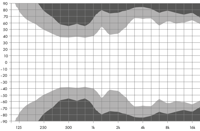
J12 horizontale Abstrahlcharakteristik 2
