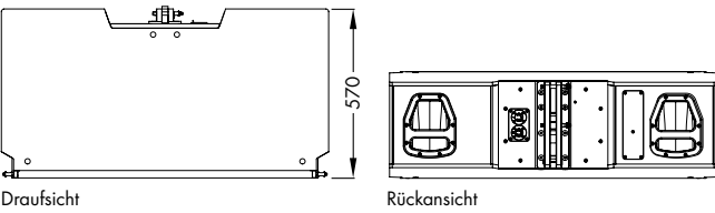
J8 und J12 Gehäuseabmessungen in mm
