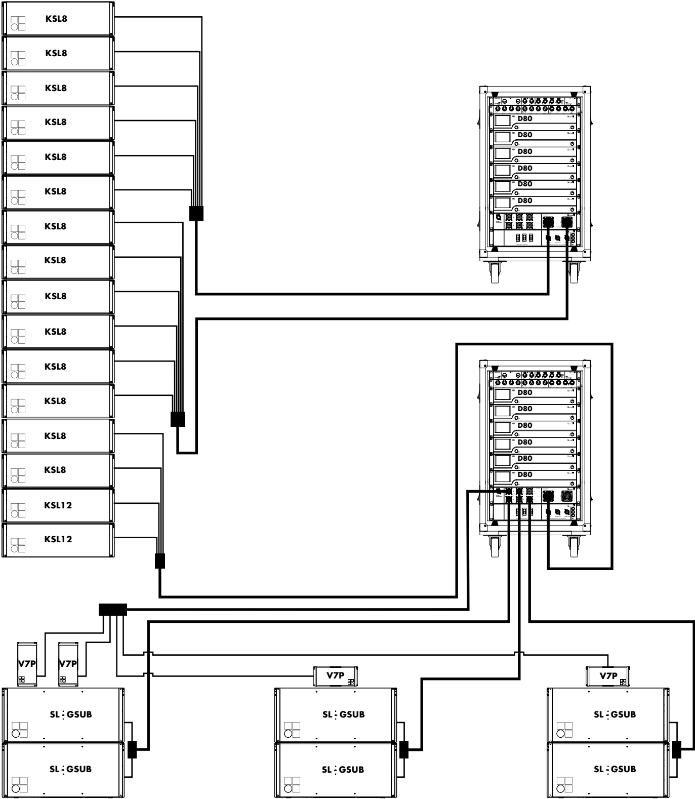
Arena Package: SL-Serie Konfiguration mit KSL8/KSL12 als Hauptarray und V7Ps als Frontfill sowie SL-GSUBs am Boden mit 6 x D80 Touring Racks
