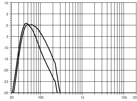
KSL-SUB/KSL-GSUB Frequenzgang, Standard- und INFRA-Modus
