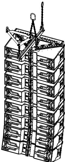
KSL8/12 Line-Array 8-tief, Tension Mode Setup - Rückansicht
