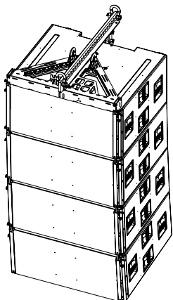
4 KSL-SUBs mit 2°-Splay-Winkeln - Vorderansicht
