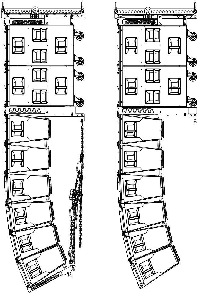
Gemischtes Array mit KSL8/12 im Compression Mode
