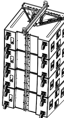
4 KSL-SUBs mit 2°-Splay-Winkeln - Rückansicht
