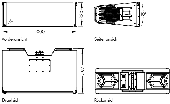
KSL8/KSL12 Gehäuseabmessungen in mm
