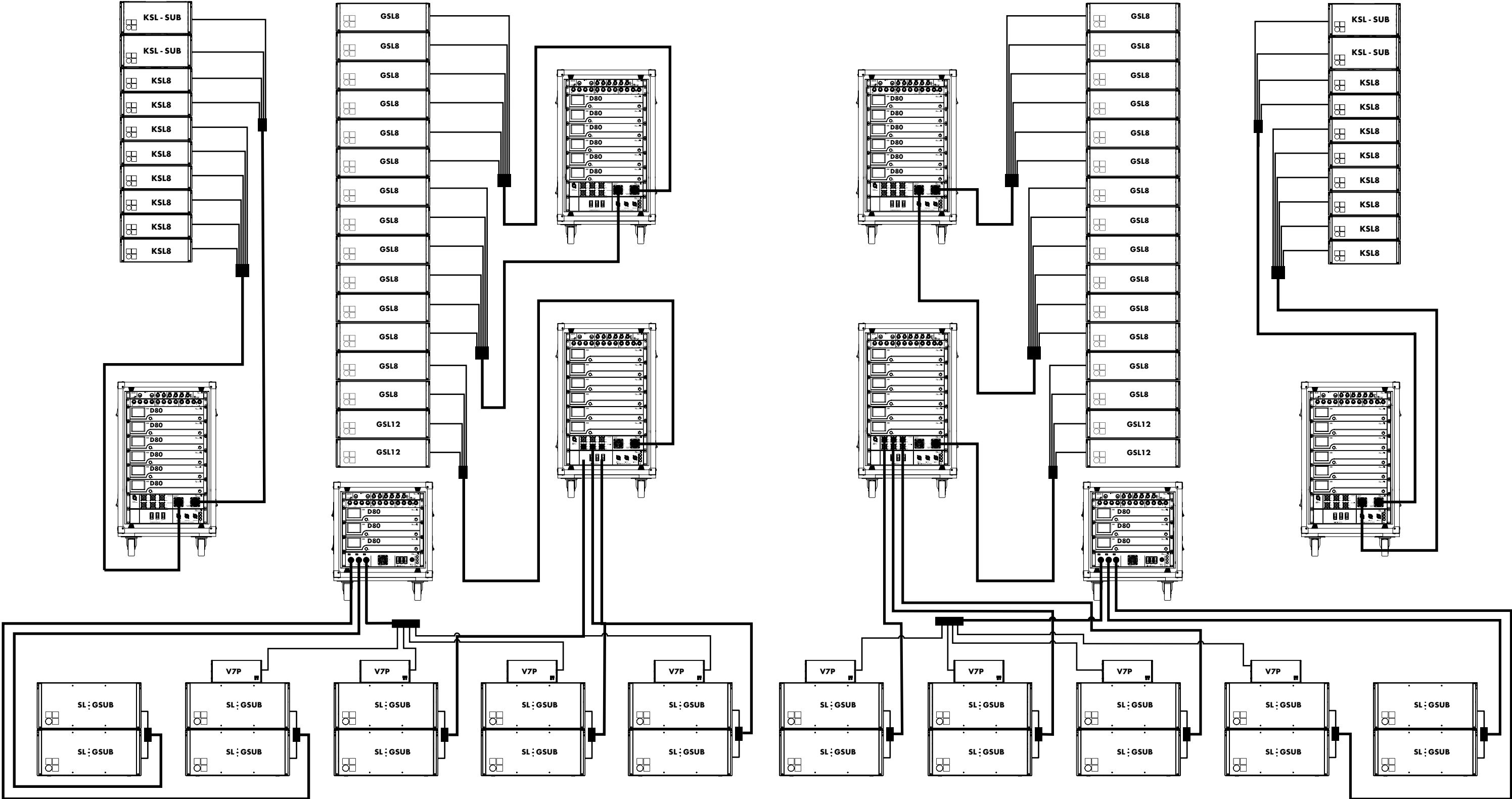
Festival Package: SL-Serie Konfiguration mit GSL8/GLS12 als Hauptarrays und KSL-SUB/ KSL8 als Outfills sowie SL-GSUBs am Boden mit 6 x D80 Touring Racks
