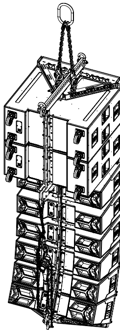
KSL-SUB/ KSL8/12 Gemischtes Array Compression Mode - Rückansicht
