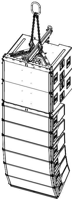
KSL-SUB/ KSL8/12 Gemischtes Array Compression Mode - Vorderansicht
