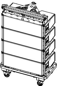
E7802 4 x KSL8/SL12 Touring Cart Beladen für Betrieb im Compression Mode mit montiertem KSL Flugrahmen und KSL Lastträger
