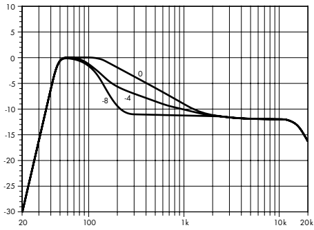
SL-CPL-Korrektur Mid 2
