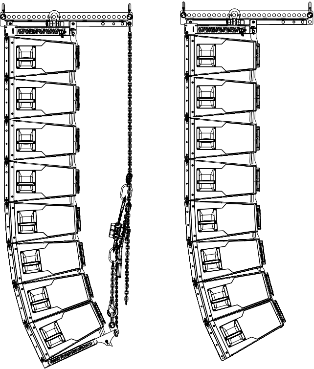
Komprimiertes KSL-Array mit Handhebelzug
