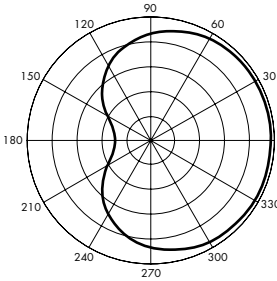
Polardarstellung, kardioid
