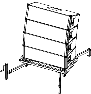
KSL8/12 Groundstack mit E7495 Touring Cart Tension und E7494 Outriggers als Groundsupport
