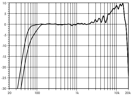
KSL12 Frequenzgang, Standard- und CUT-Modus 1
