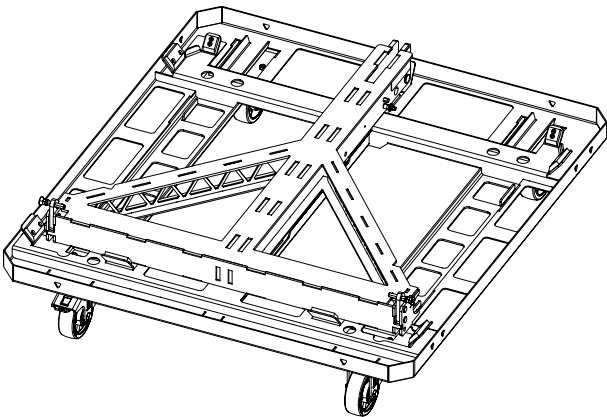
E7804 Touring Cart KSL-SUB/KSL-GSUB mit KSL-SUB Adapterrahmen 1
