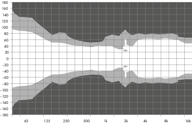
KSL12 horizontale Abstrahlcharakteristik²
