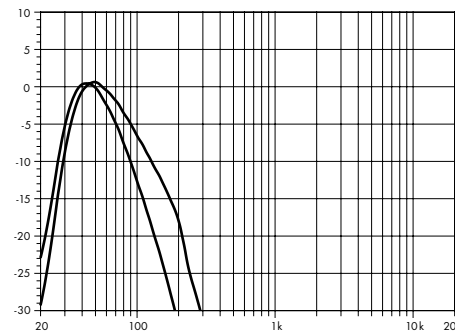
SL-SUB/SL-GSUB Frequenzgang, Standard- und INFRA-Modus
