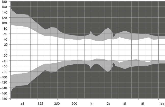
KSL8 horizontale Abstrahlcharakteristik²
