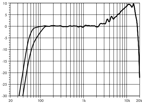
KSL8 Frequenzgang, Standard- und CUT-Modus 1
