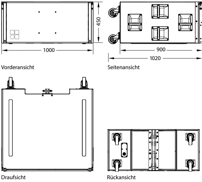
KSL-SUB/KSL-GSUB Gehäuseabmessungen in mm
