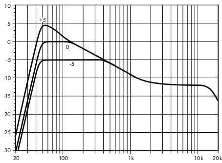
SL-CPL-Korrektur Low 2
