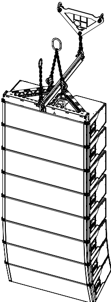
KSL8/12 Line-Array 8-tief, Tension Mode Setup - Vorderansicht
