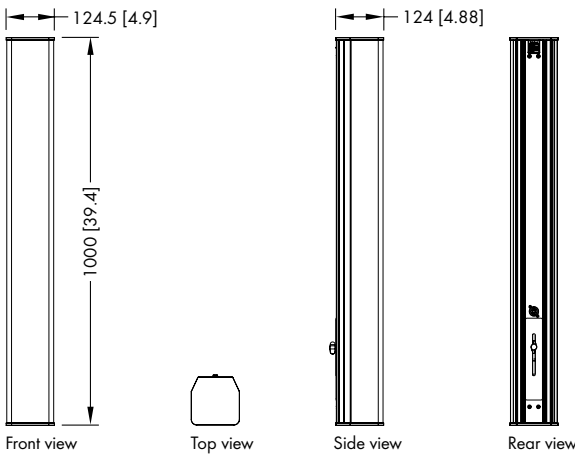
24C キャビネット寸法mm[インチ]
