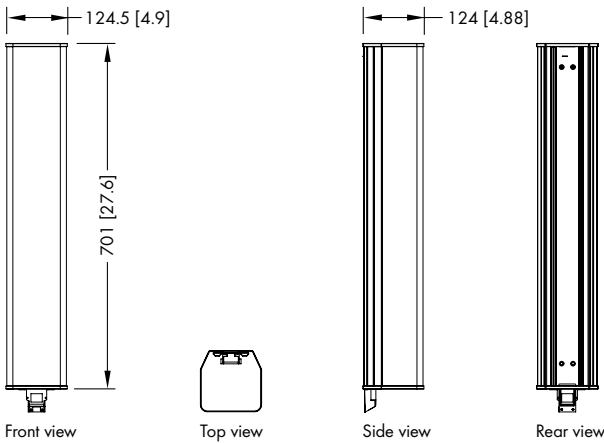
24C-E キャビネット寸法mm[インチ]
