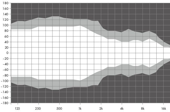
24C 水平指向特性 2
