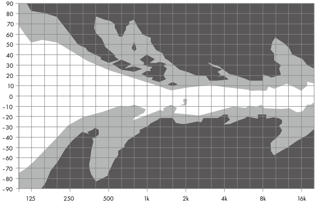
24C と24C-Eの併用時の垂直指向特性 2
