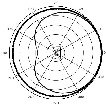
無響音場で水平ボーラープロット、一般的なコラムラウドスピーカーとカーディオイドラウドスピーカーの対比
