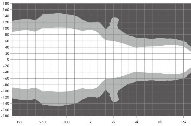
16C 水平指向特性 2
