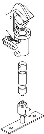
Kugelgelenk E3 mit TV-Zapfen und Rohrkralle
