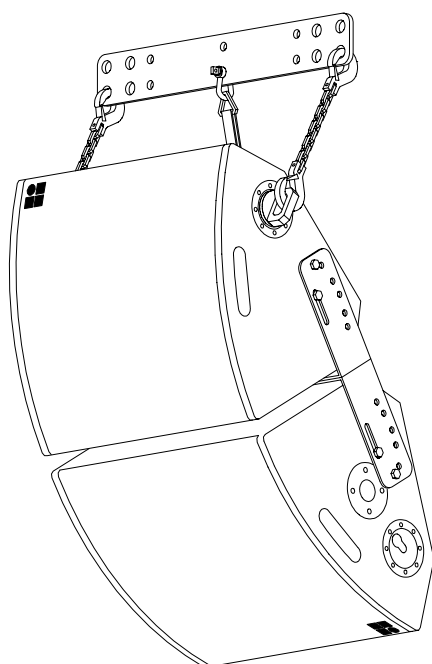
MAX-Array mit Querbügeln und C4-Riggingzubehör
