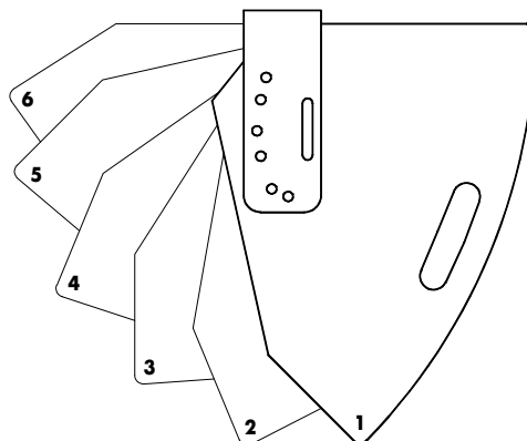
Winkleinstellungen des Querbügels
