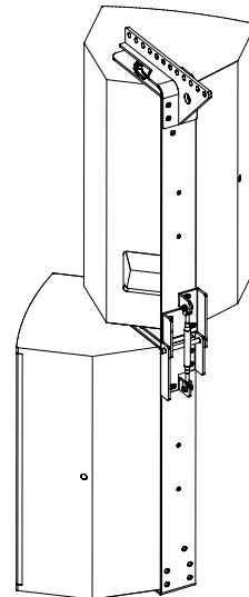
Line-Array mit individueller horizontaler Ausrichtung mit: Z5051 Querbügel Ci60/Ci90 Z5053 Gelenkverbinder Ci60/Ci90 und Z5054 Flugadapter Ci60/Ci90
