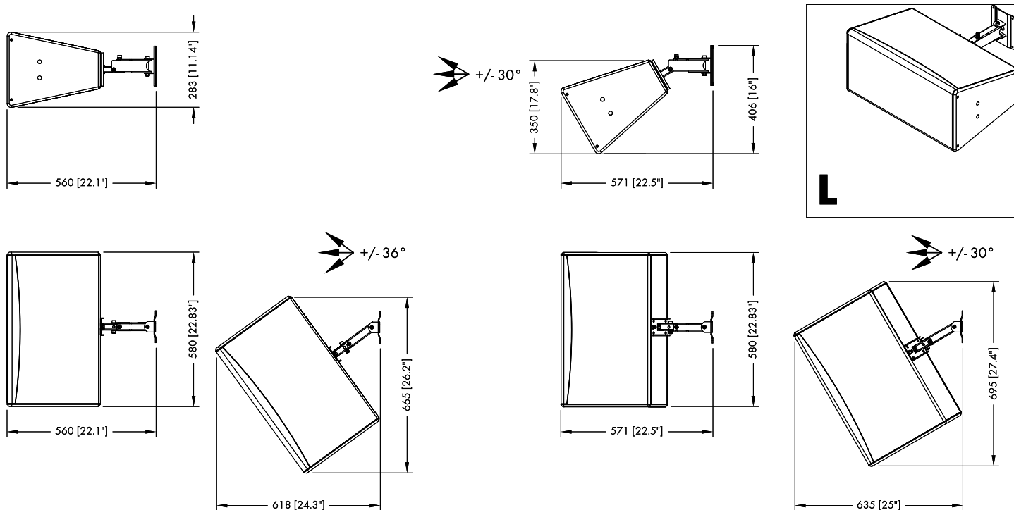
Z5403 Wandhalterung L, Einbaumaße in mm [Zoll], 10S/10S-D horizontale Montage
