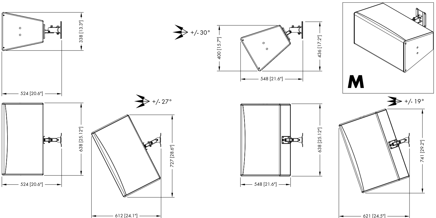
Z5402 Wandhalterung M, Einbaumaße in mm [Zoll], 12S/12S-D horizontale Montage
