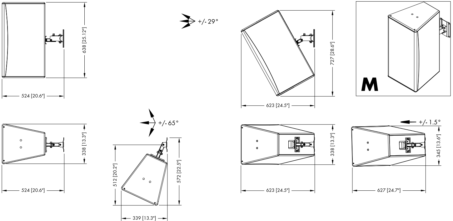
Z5402 Wandhalterung M, Einbaumaße in mm [Zoll], 12S/12S-D vertikale Montage
