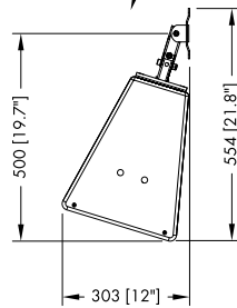
Z5402 Wandhalterung M, Einbaumaße in mm [Zoll], 10S/10S-D vertikale Montage
