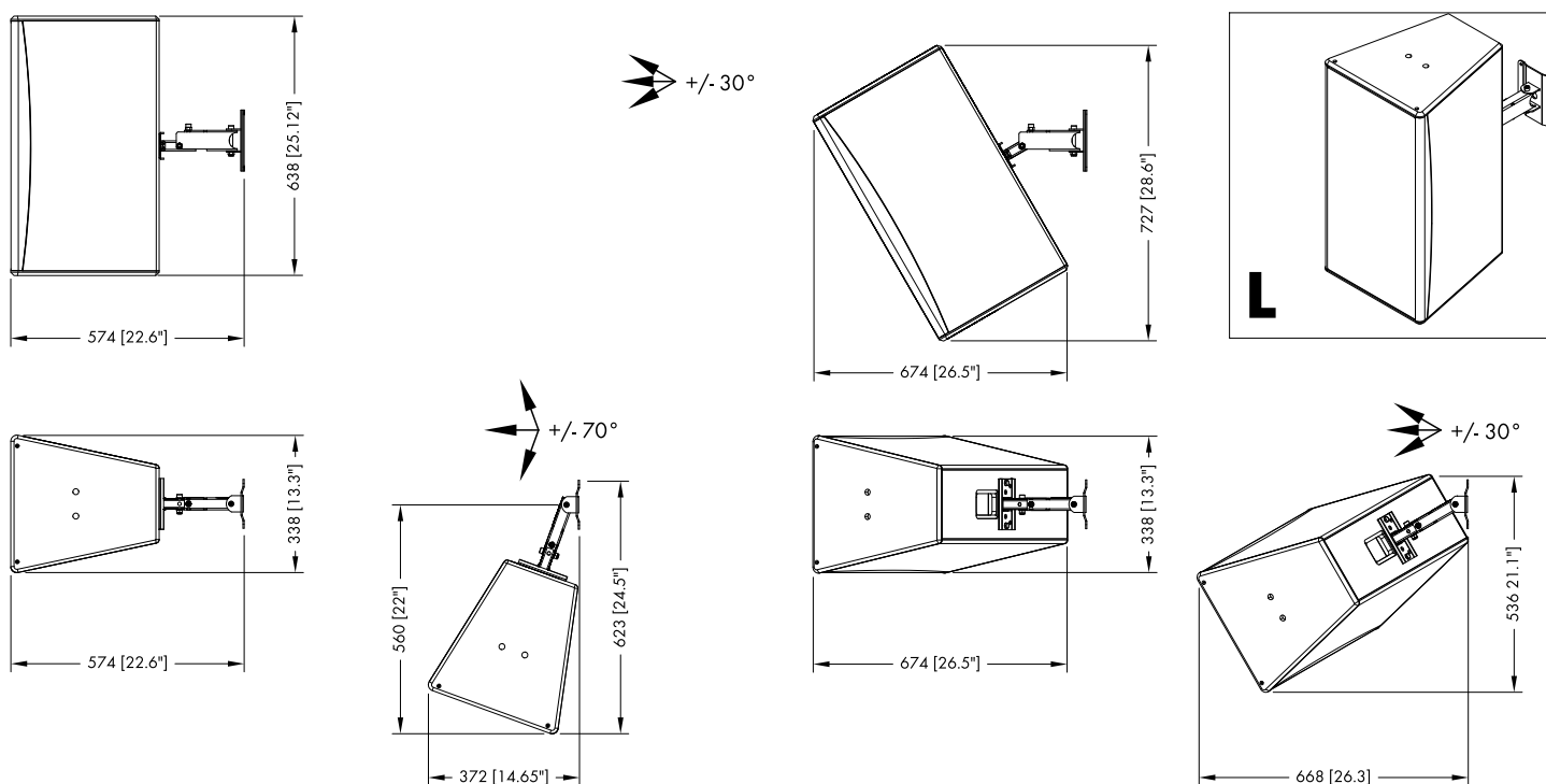
Z5403 Wandhalterung L, Einbaumaße in mm [Zoll], 12S/12S-D vertikale Montage
