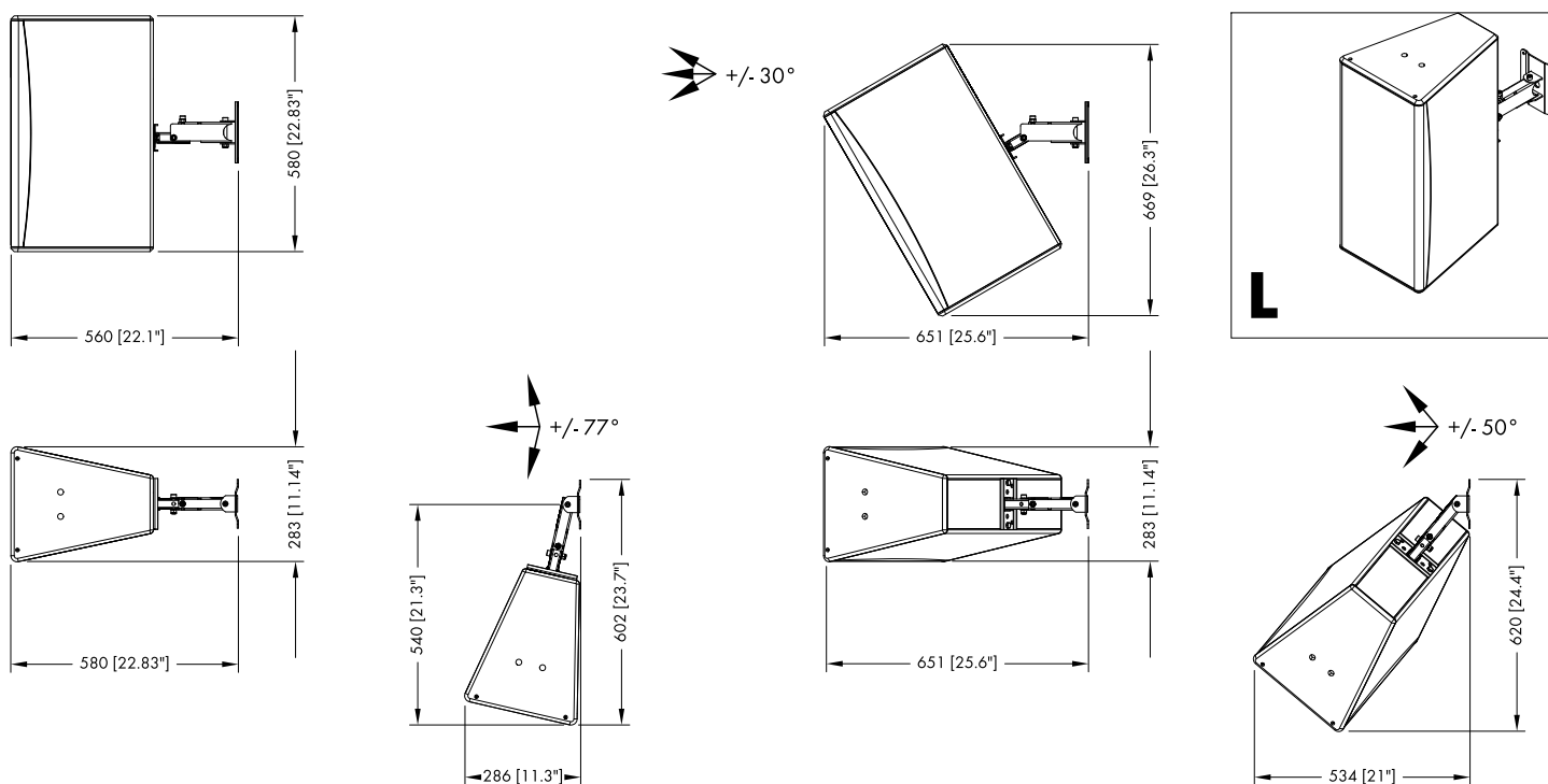
Z5403 Wandhalterung L, Einbaumaße in mm [Zoll], 10S/10S-D vertikale Montage
