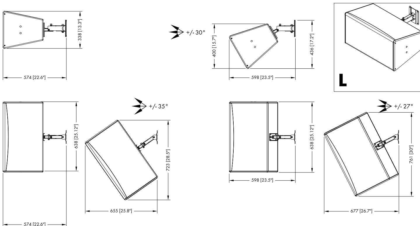
Z5403 Wandhalterung L, Einbaumaße in mm [Zoll], 12S/12S-D horizontale Montage
