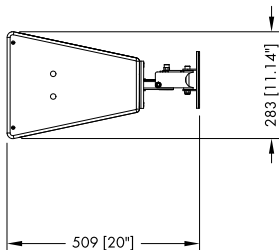
Z5402 Wandhalterung M, Einbaumaße in mm [Zoll], 10S/10S-D vertikale Montage
