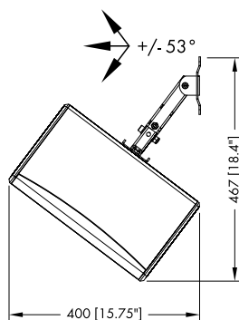
Z5403 Wandhalterung L, Einbaumaße in mm [Zoll], 85 horizontale Montage
