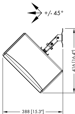
Z5402 Wandhalterung M, Einbaumaße in mm [Zoll], 85 horizontale Montage
