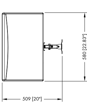
Z5402 Wandhalterung M, Einbaumaße in mm [Zoll], 10S/10S-D horizontale Montage
