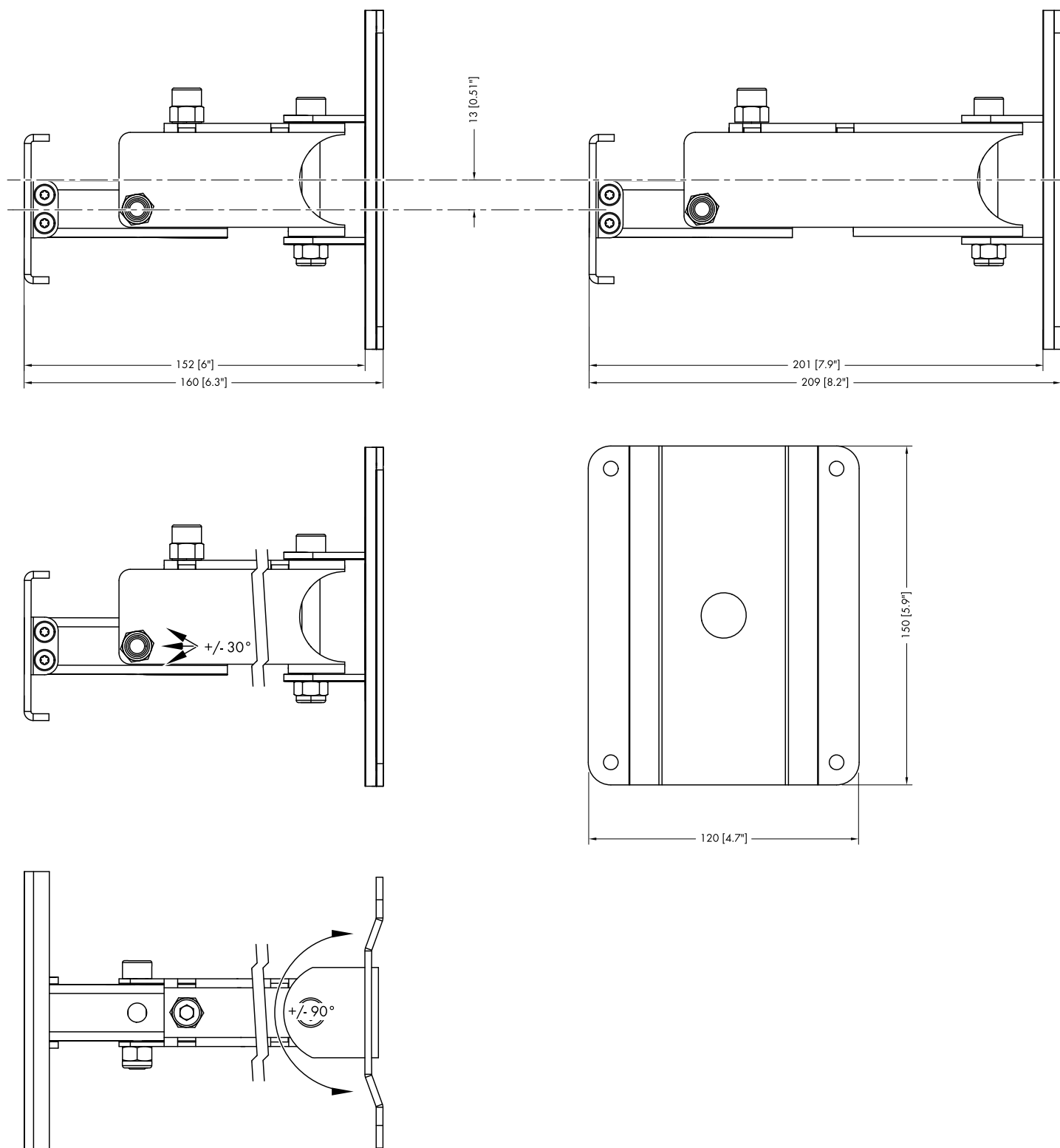
Z5402/03 Wandhalterung M/L Abmessungen in mm [Zoll]
