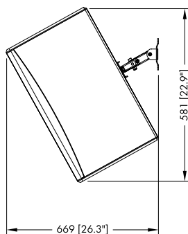
Z5402 Wandhalterung M, Einbaumaße in mm [Zoll], 10S/10S-D horizontale Montage
