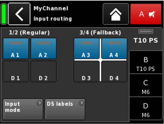
フォールバック設定の例 A1/A2 Regular、A3/A4 Fallback。 フォールバック入力がアクティブ。
