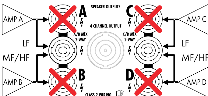
2 x 2-Way Active モード
