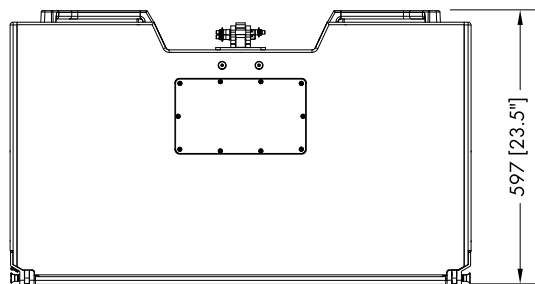
Dimensions de l'enceinte KSL8/KSL12 en mm [pouces]
