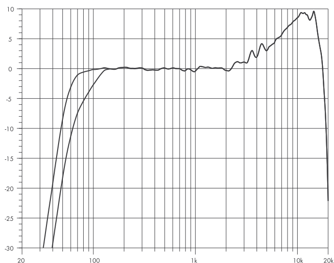
KSL8: Réponse en fréquence*, modes standard et CUT
