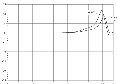
Correction de la réponse en fréquence de la fonction HFC* *diagramme schématique
