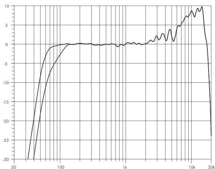
KSL12: Réponse en fréquence*, modes standard et CUT
