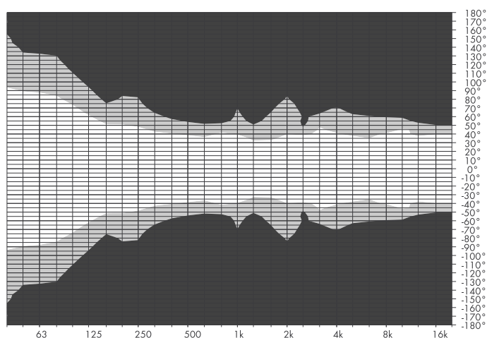
Diagramme isobare horizontal KSL8
