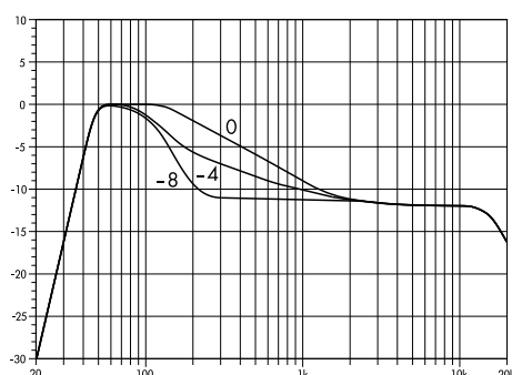
Correction de la réponse en fréquence de la fonction Coupling pour les graves et les bas-médiums*
