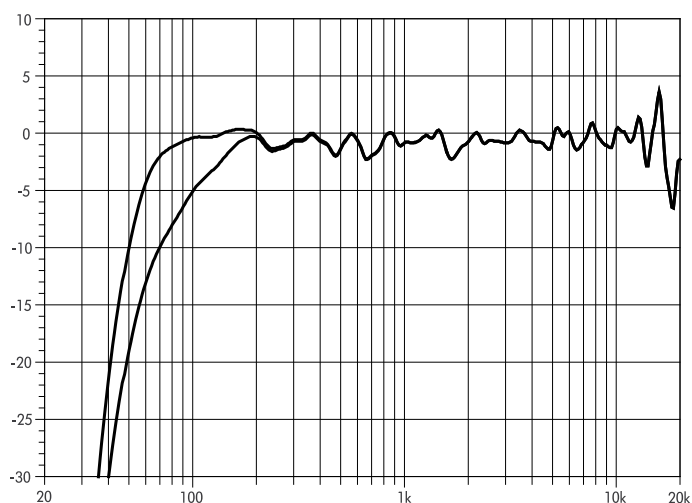
Fig. 17 : Réponse en fréquence de la 10S, modes standard et CUT
