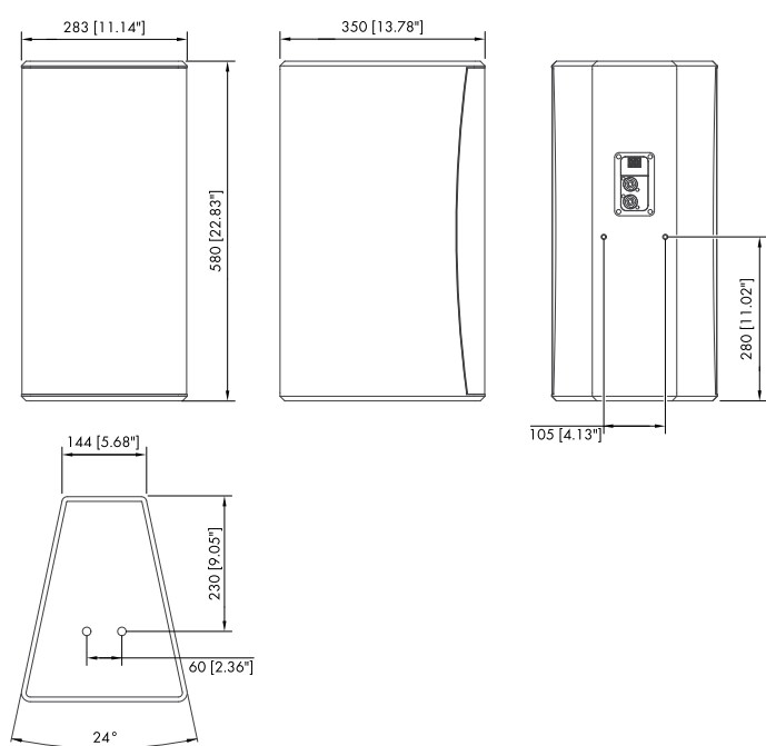
Fig. 19 : Dimensions de l'enceinte 10S/10S-D en mm [pouces]
