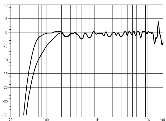
Fig. 18 : Réponse en fréquence de la 10S-D, modes standard et CUT
