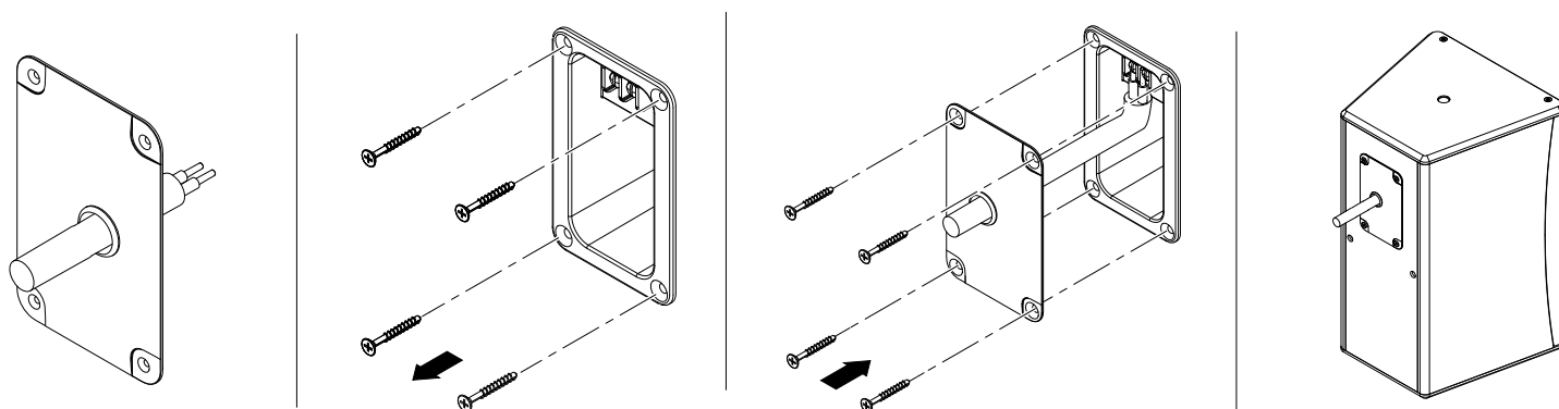
Fig. 4 : Raccordement par câble fixe
