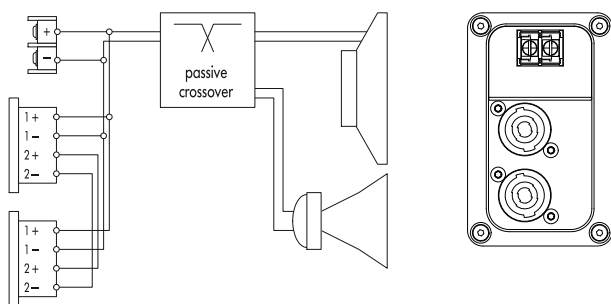
Verdrahtung der Anschlussbuchsen
