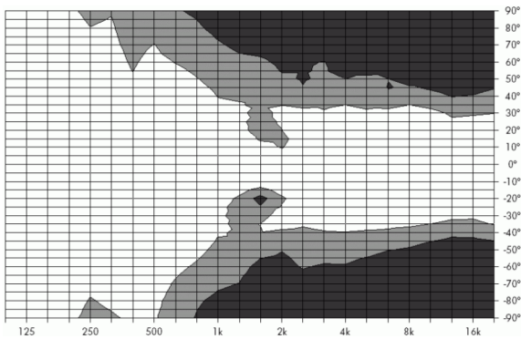
Abb. 9: Abstrahlcharakteristik horizontal
