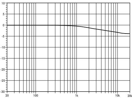
Abb. 5: Frequenzgangkorrektur der HFA-Schaltung
