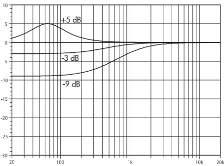
Abb. 6: Frequenzgangkorrektur der CPL-Schaltung
