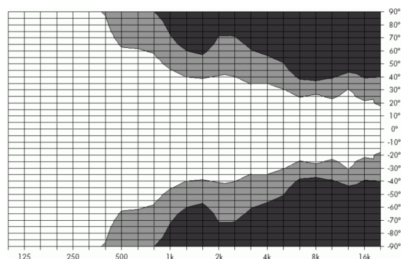
Abb. 14: Abstrahlcharakteristik vertikal
