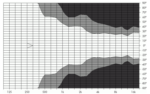
Abb. 10: Abstrahlcharakteristik vertikal
