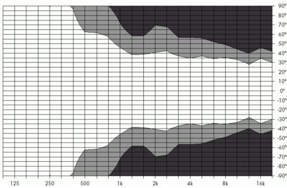
Abb. 7: Abstrahlcharakteristik horizontal
