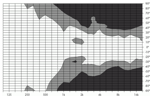
Abb. 12: Abstrahlcharakteristik vertikal
