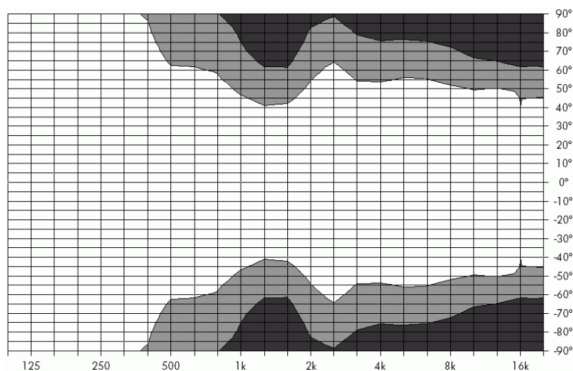
Abb. 11: Abstrahlcharakteristik horizontal
