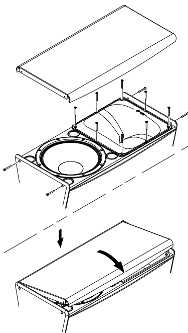
Abb. 15: Drehen des Hochttonhorns
