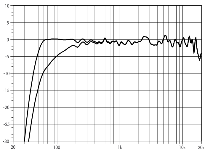
Abb. 16: 12S Frequenzgang, Standard und CUT-Modus
