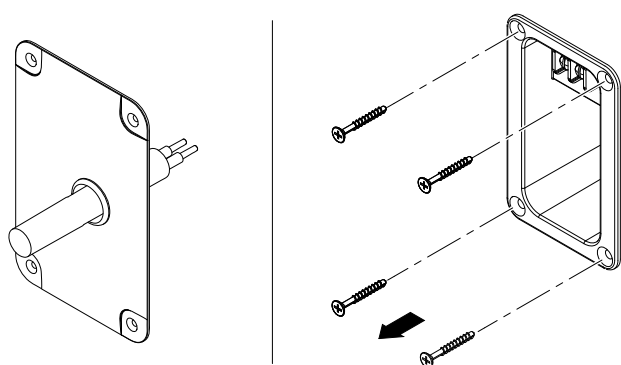
Abb. 3: Festanschluss
