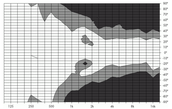
Abb. 8: Abstrahlcharakteristik vertikal
