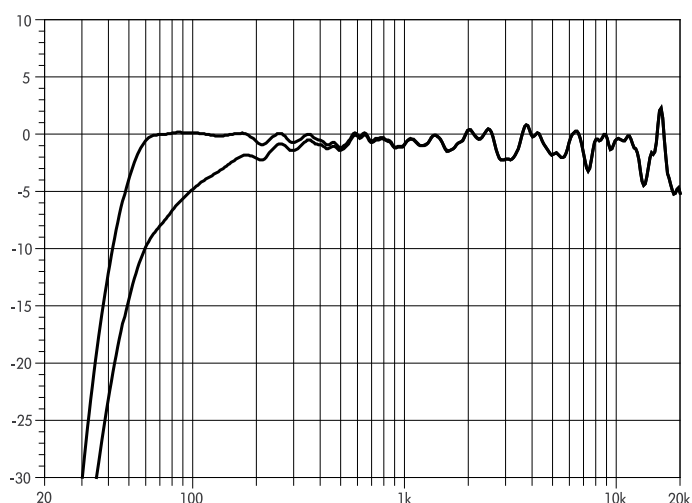
Abb. 17: 12S-D Frequenzgang, Standard und CUT-Modus
