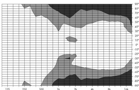
Abb. 13: Abstrahlcharakteristik horizontal
