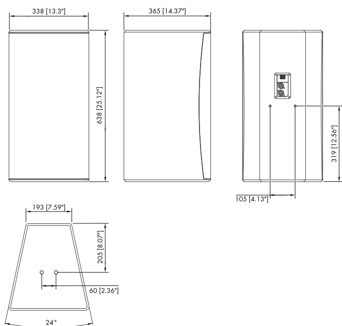
Abb. 18: 12S/12S-D Gehäuseabmessungen in mm [Zoll]
