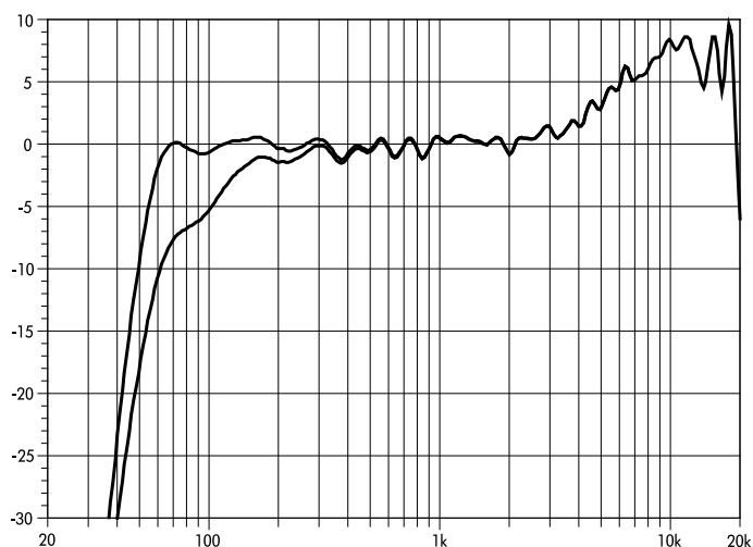
Yi8 Frequenzgang, Standard und CUT-Modus
