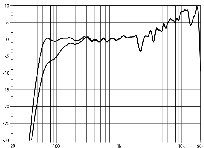
Yi12 Frequenzgang, Standard und CUT-Modus
