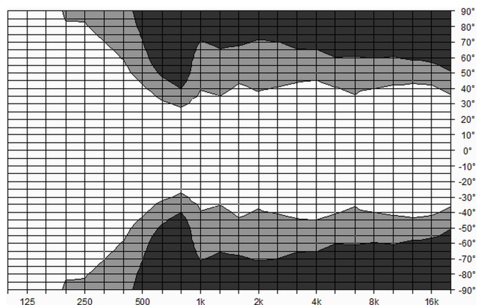
Abstrahlcharakteristik Yi8 horizontal
