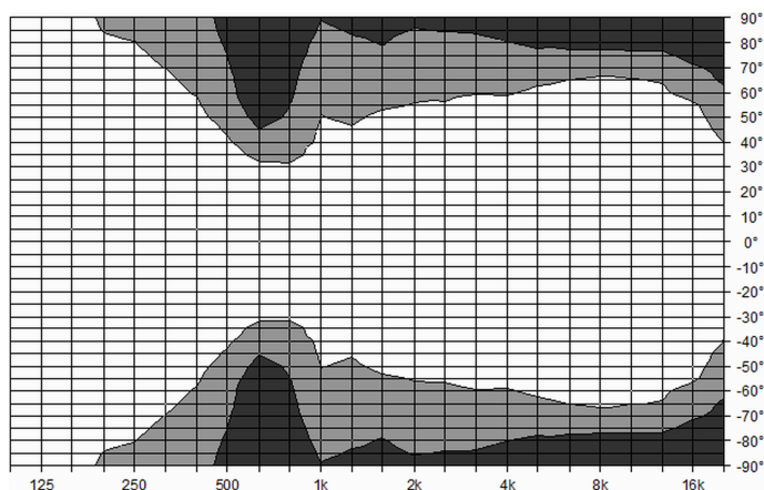
Abstrahlcharakteristik Yi12 horizontal
