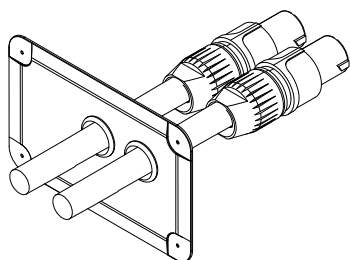
NL4-Anschluss mit Abdeckplatte [1]
