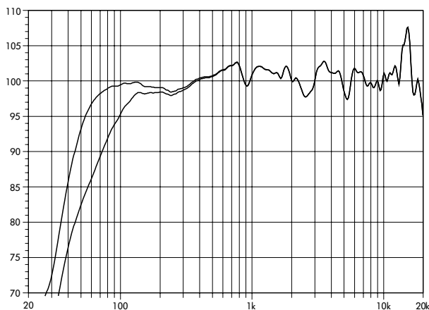
MAX Frequenzgang (MAX Setup, Bodenkopplung), Standard und CUT-Schaltung
