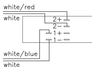
Fig. 2: 4-adriger Betrieb NL4
