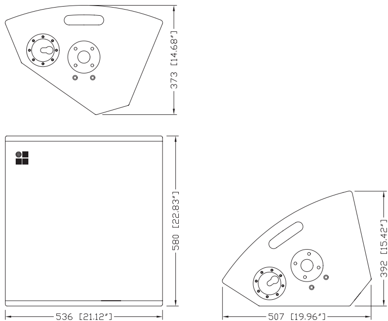
Gehäuseabmessungen MAX in mm [Zoll]
