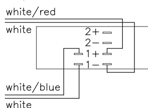
Fig. 1: 2-adriger Betrieb NL4
