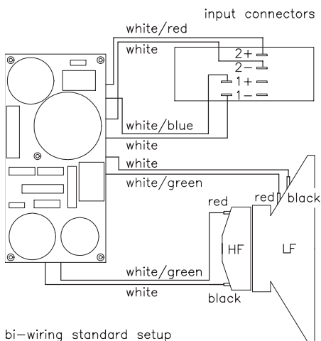
Verdrahtungsschema MAX (Standard: 4-adriger Betrieb NL4)
