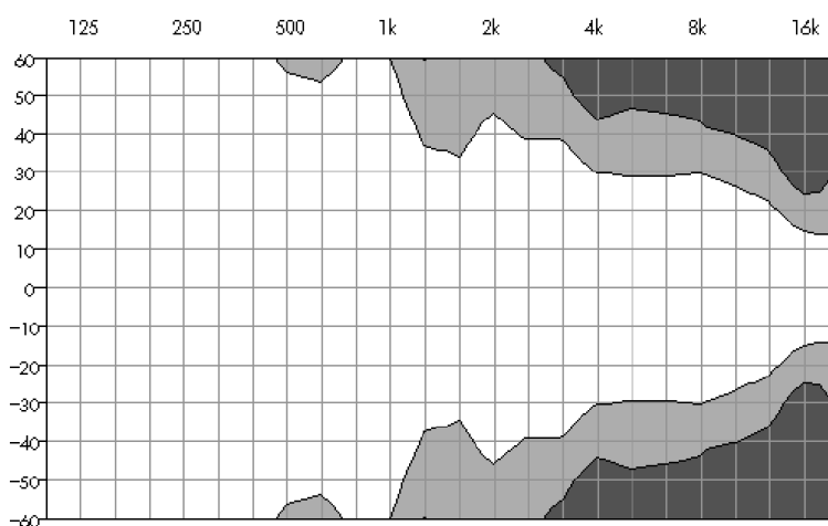
Isobarendiagramm MAX
