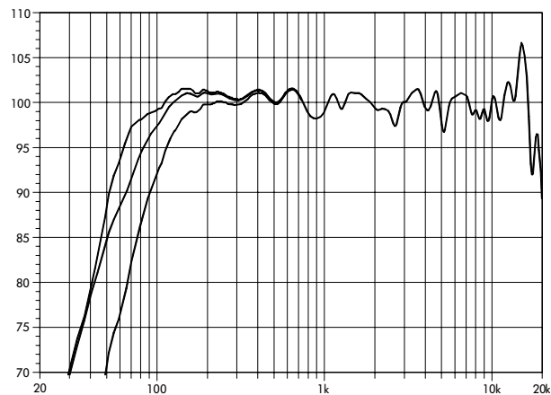
MAX Frequenzgang (LINEAR Setup, Freifeld) CPL +5, Standard und CUT-Schaltung
