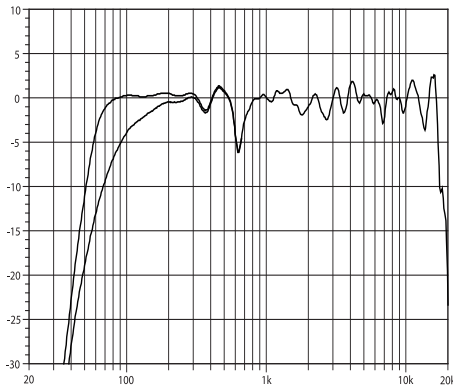
Fig. 9: Respuesta de frecuencia de Qi7, estándar y ajustes de CUT
