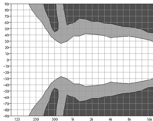
Fig. 7: Diagrama de isóbara Qi7 horizontal, configuración horizontal con la trompeta girada
