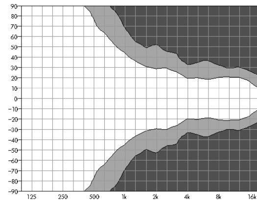
Fig. 8: Diagrama de isóbara Qi7 vertical, configuración horizontal con la trompeta girada
