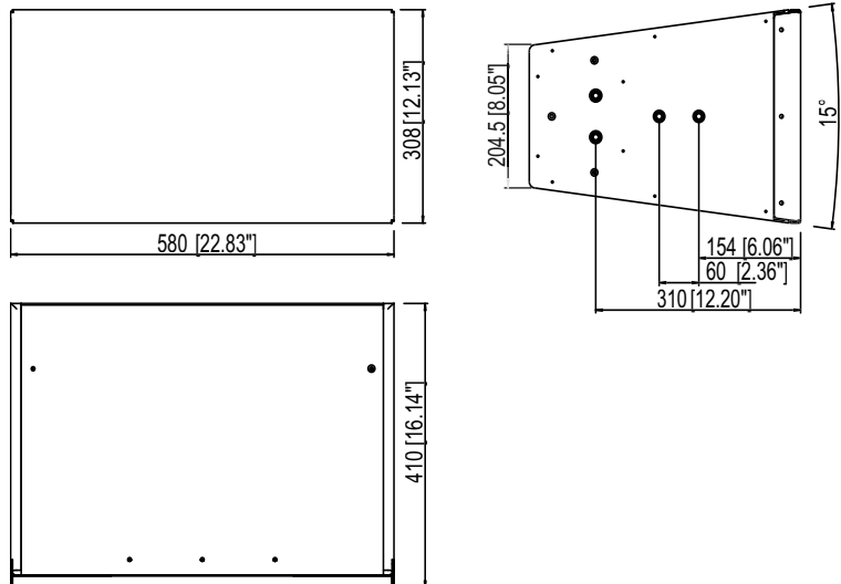
Fig. 10: Dimensiones de la caja Qi7 en mm [pulgadas]
