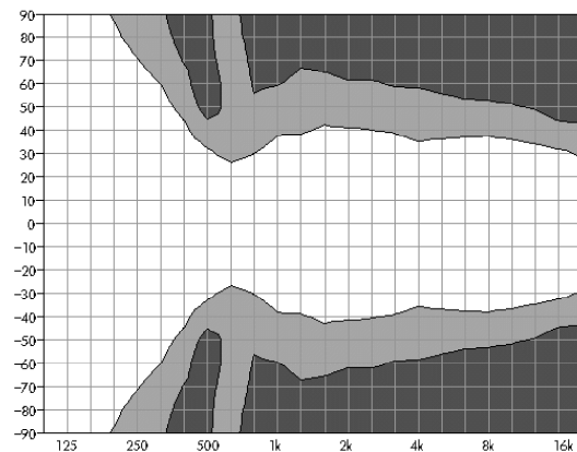
Fig. 7: Diagramme isobare Qi7 horizontal, configuration horizontale avec pavillon tourné
