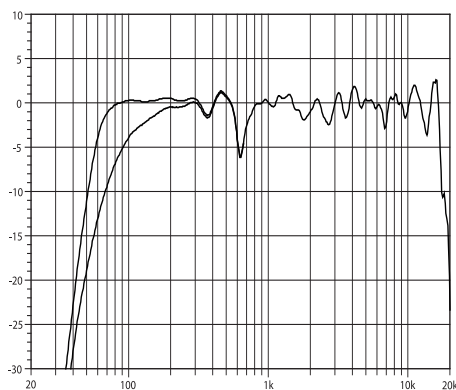
Fig. 9: Réponse en fréquence de la Qi7, modes standard et CUT
