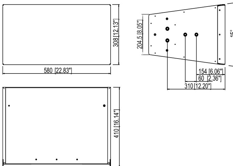
Fig. 10: Qi7 dimensions du coffre en mm [inch]
