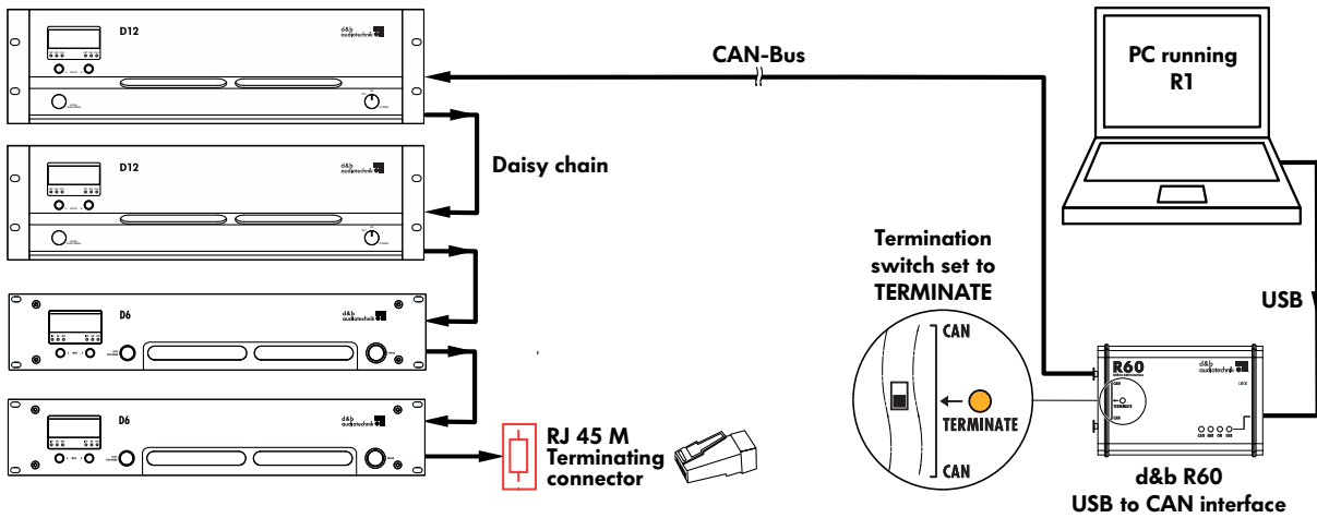
Beispiel 1: Einfaches Netzwerk aus d&b Verstärkern mit terminiertem Interface am "Beginn" des CAN-Bus-Segments.
