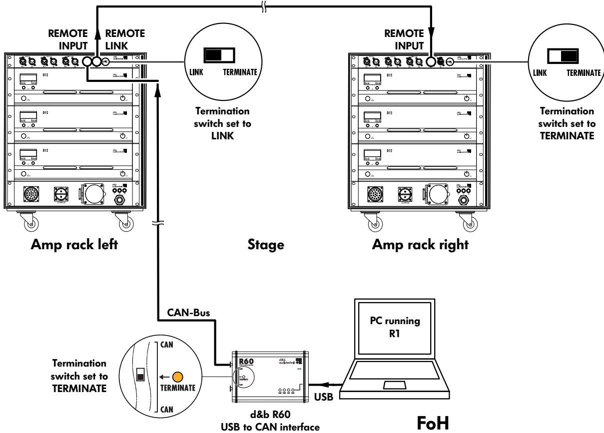
Beispiel 4: Gleicher Netzwerkaufbau wie in Bsp. 3, gezeigt mit Touringracks (Z5310) und die Stellung der Terminierungsschalter der I/O-Panels (Z5313).
