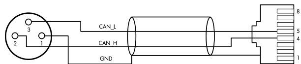
Fig. 9: CAN Adapterkabel XLR auf RJ 45 M
