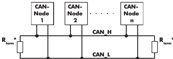
Fig. 5: Physikalischer CAN-Bus
