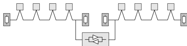
Fig. 3: Repeater zur Verbindung zweier Bus-Segmente
