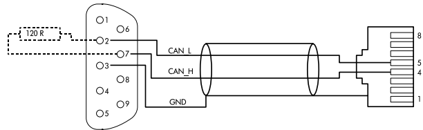
Fig. 8: CAN Adapterkabel D-SUB-9 auf RJ 45 M
