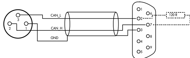
Fig. 10: CAN Adapterkabel XLR auf D-SUB 9 F
