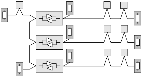
Fig. 4: Repeater zur Sternverkabelung
