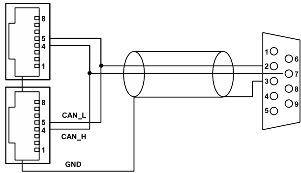
Fig. 7: Z6117.000 D-SUB 9 F auf 2 x RJ 45 F CAN Adapter
