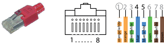
Fig. 6: RJ 45 Stecker mit Metallgehäuse (CAN Masse) Pin 1 Indikation (Stecker Frontansicht) und Farbcode gemäß T568B Standard
