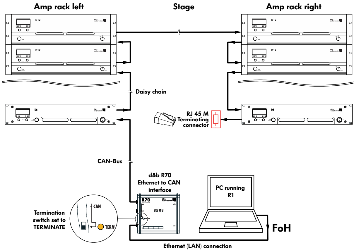
Beispiel 3: Typisches Stereo Setup mit Überwachung und Steuerung vom FoH-Platz
